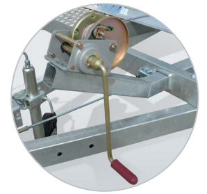
Seilwinde mit Halter ist optional
